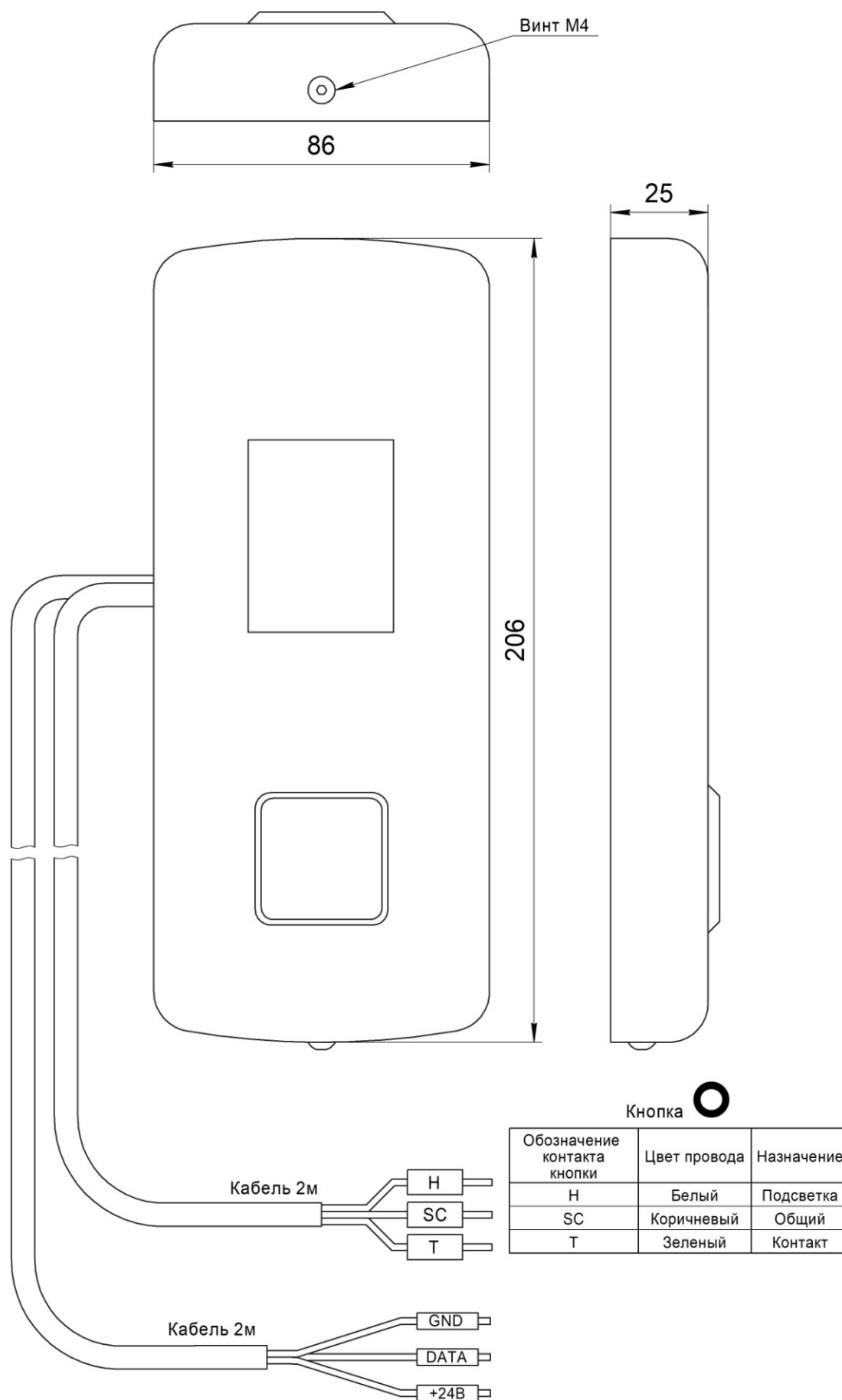
Рис.1 Внешний вид и габаритные размеры Вызывного поста ВП-1000-1074-27
